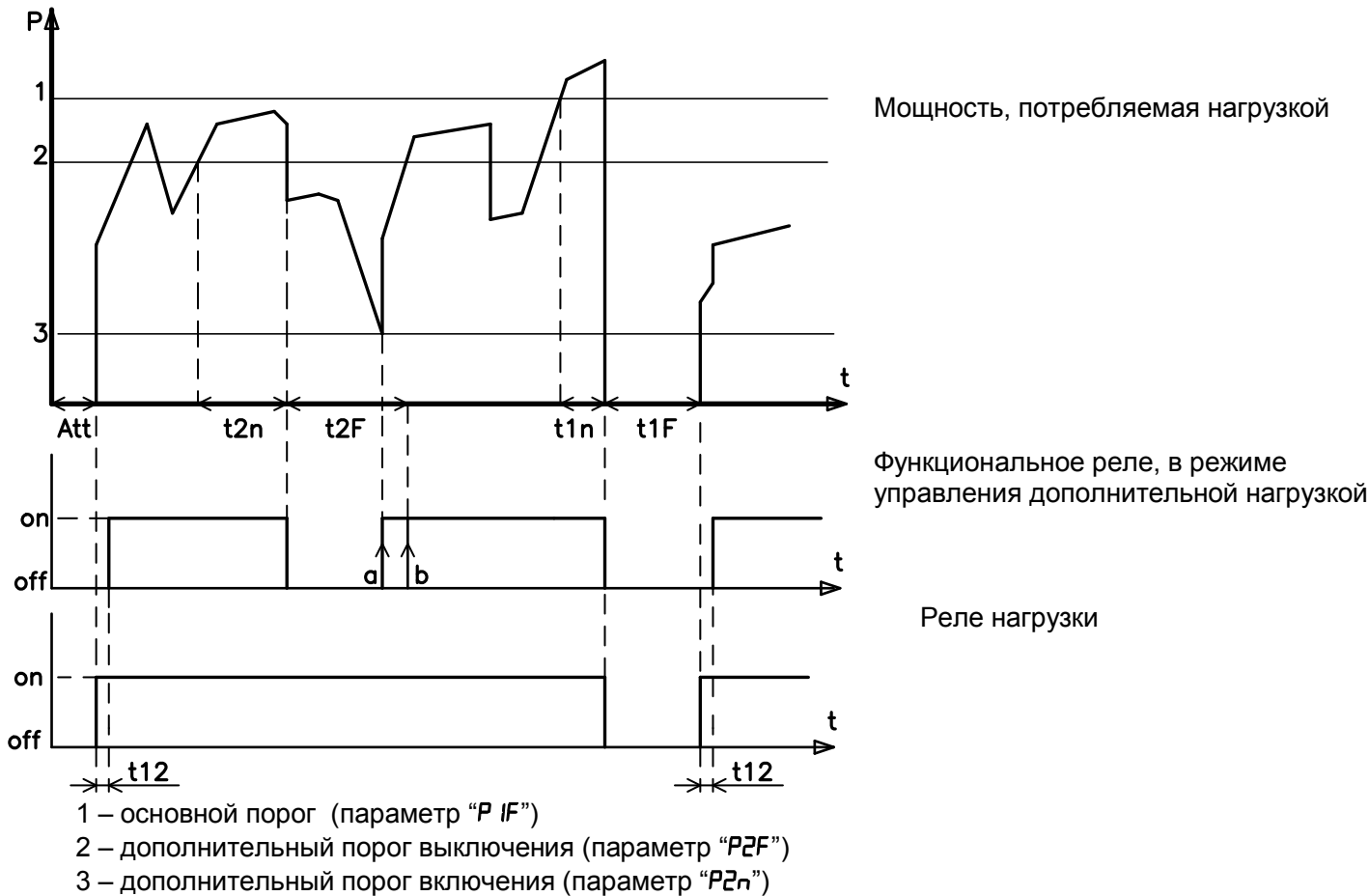
Рисунок 1.3 - Работа OM-310 в режиме ограничения мощности при r5=2
