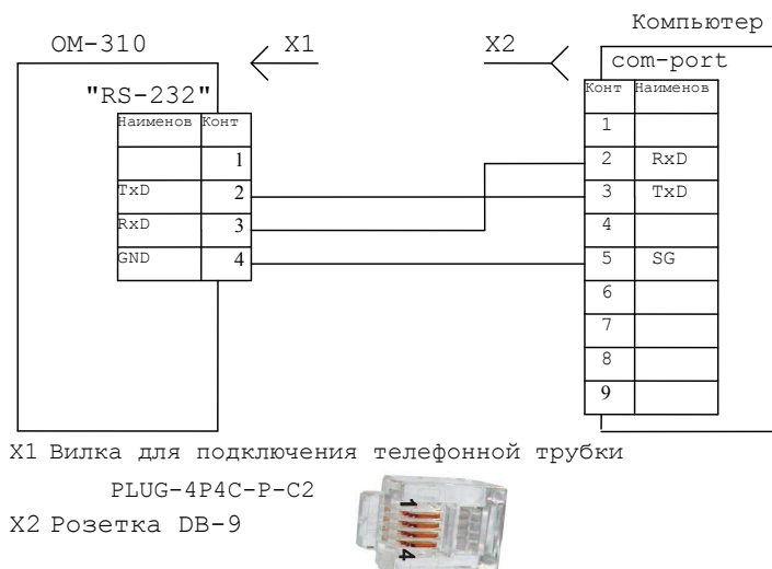
Рисунок 2.2 - Схема подключения ОМ-310 к компьютеру
